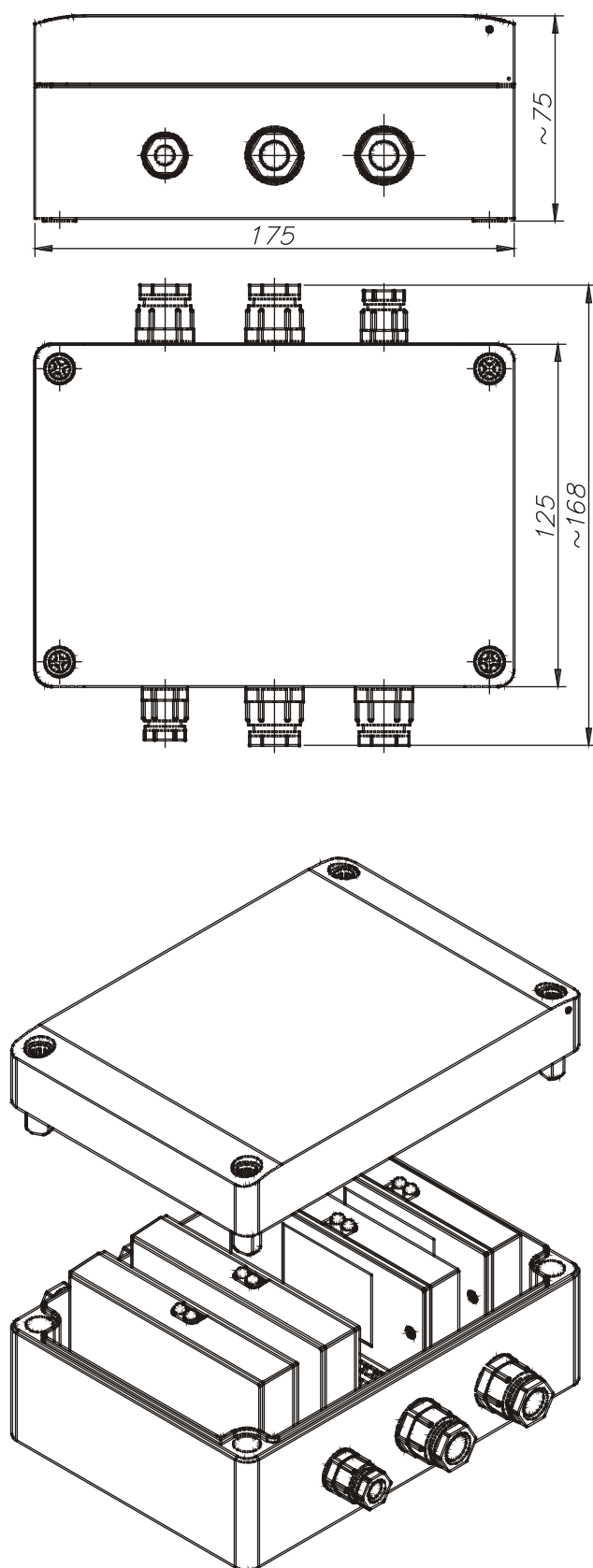
Rys. 4 Wymiary obudowy 4xEKS
