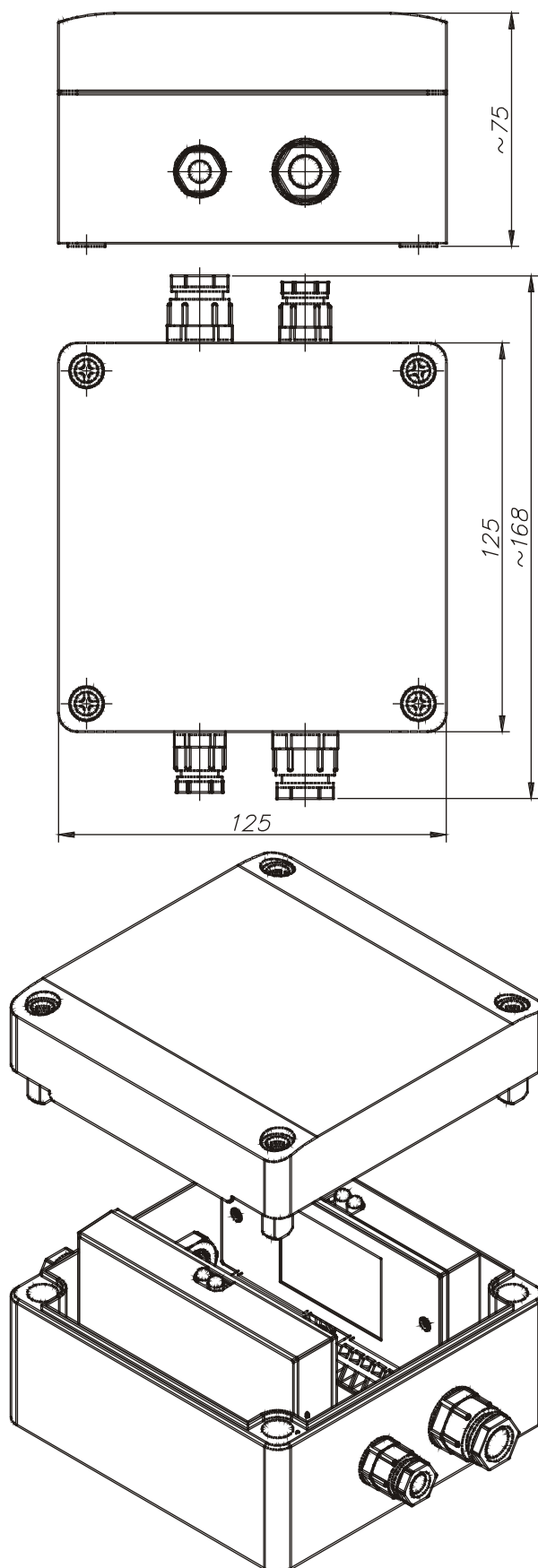
Rys.3 Wymiary obudowy 2xEKS
